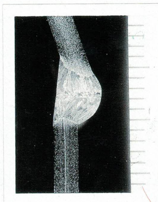
Test No.1C (Pos.90°) - G X 6 Etching: Aqua Regia
