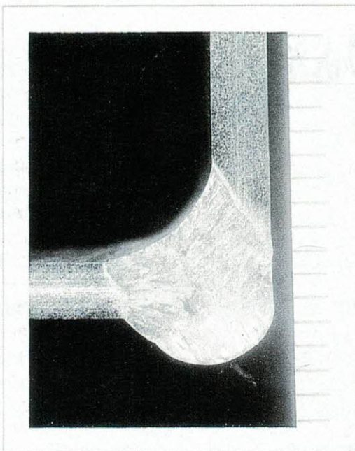
Test No.1C (Pos.0°) - G X 6 Etching: Aqua Regia
